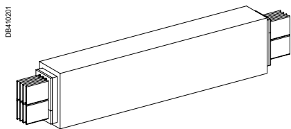
FT - Огнестойкая прямая секция
